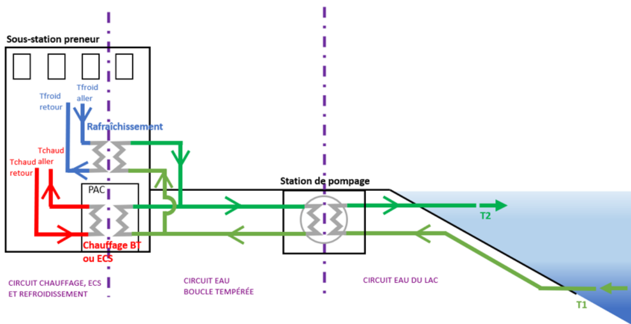
Schéma de principe du captage d'eau du lac à Evian-les-Bains Bord du Lac
